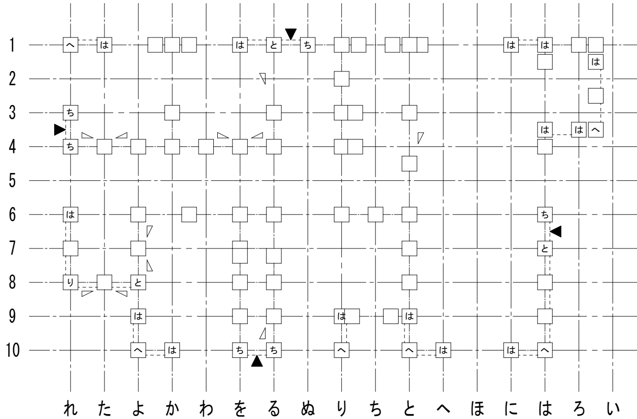
1 階柱壁伏図
